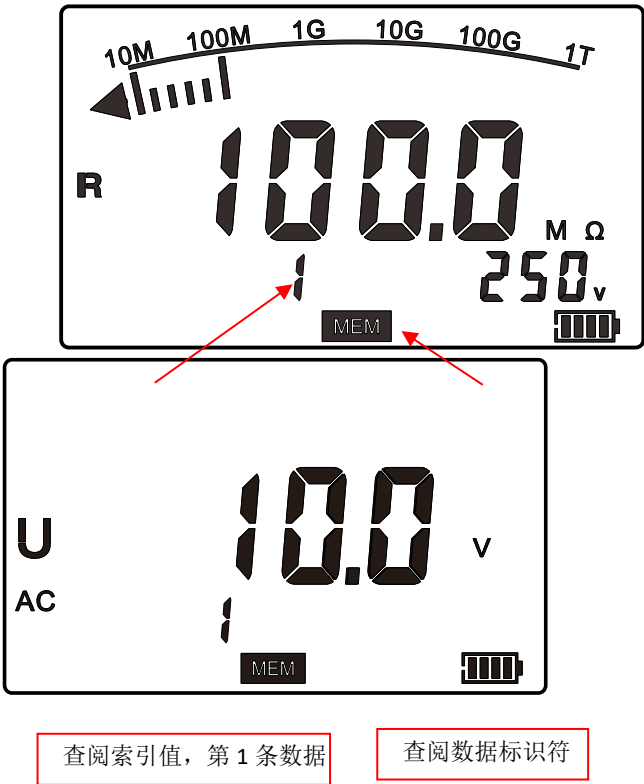
图 13-1 电阻查阅
