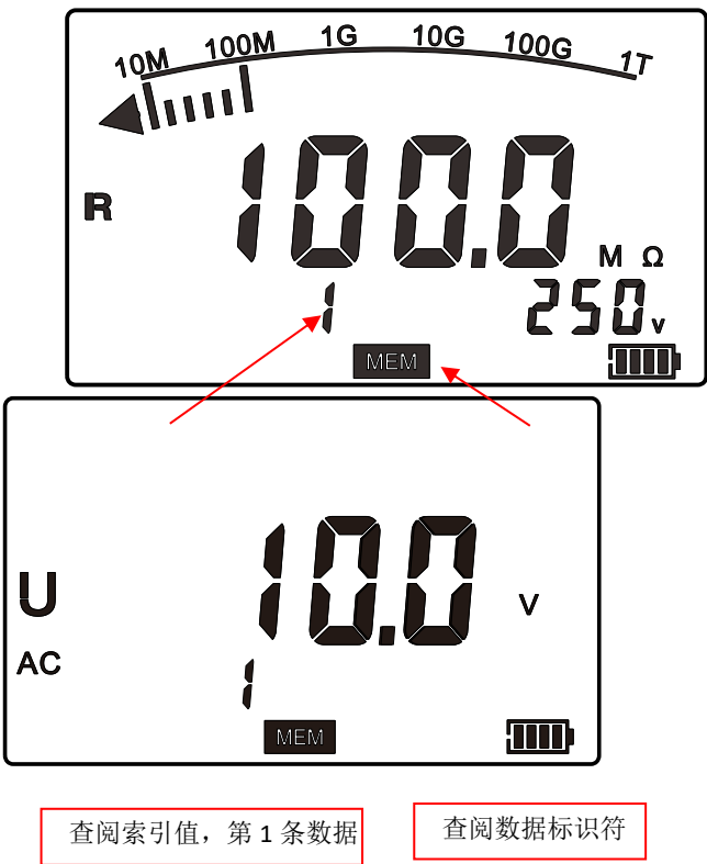
图 13-1 电阻查阅
