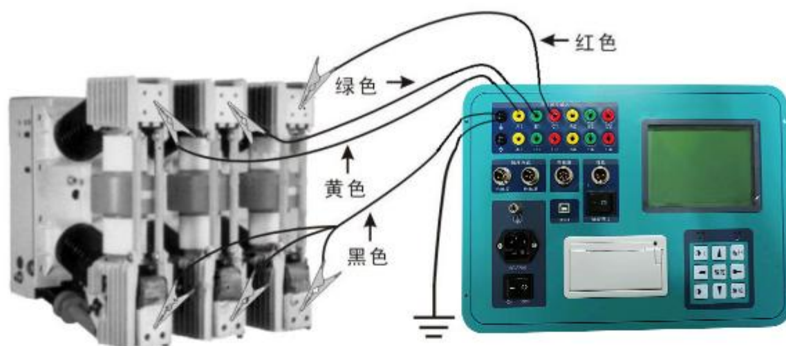
断口接线图（三断口）
