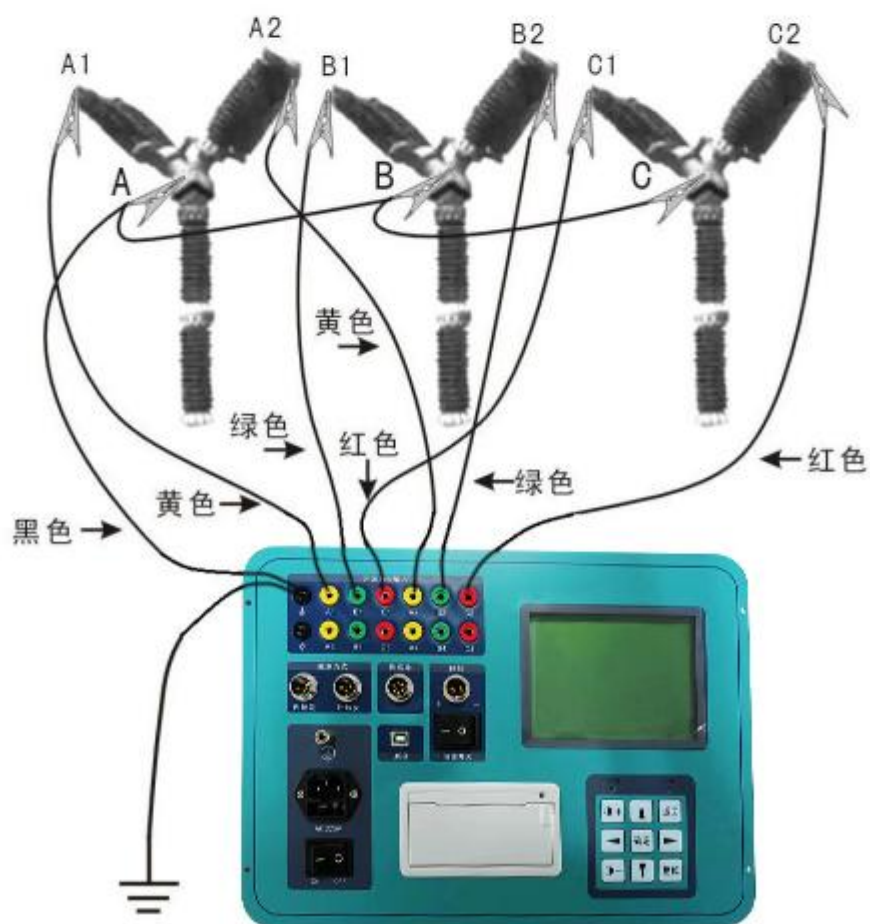
断口接线图（六断口）
