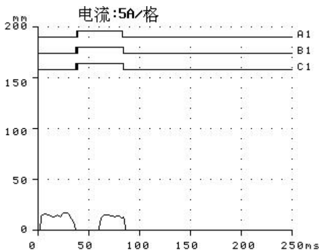
合一分闸测试图形
