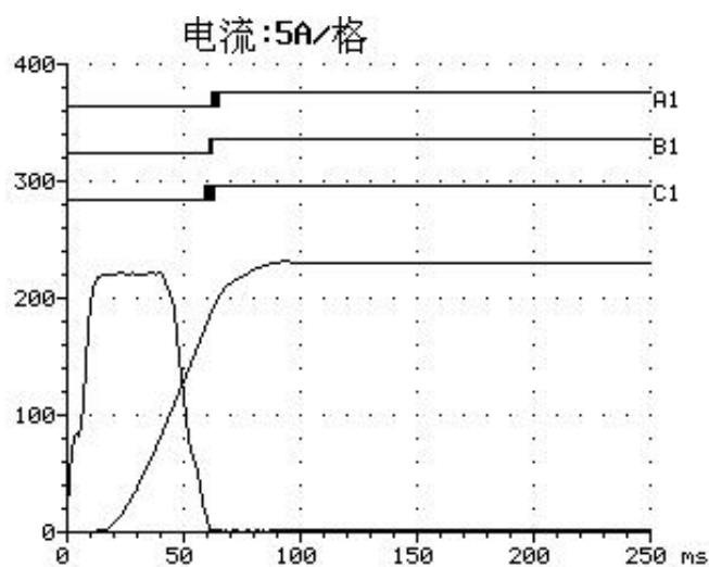
分闸测试图形
