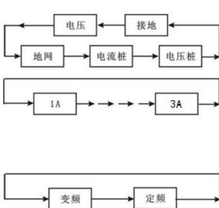
图 10 参数设定流程图
