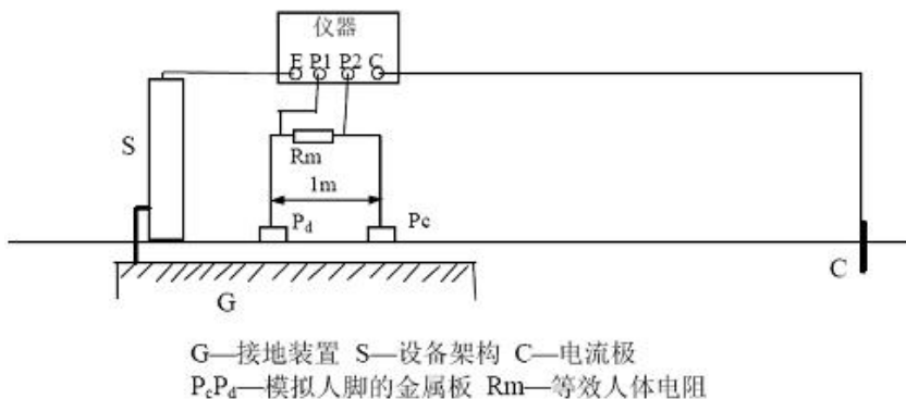
图6 跨步电压测量接线图
