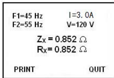
图 12 测量结果显示
