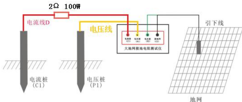
图 2：串入电阻后现场试验图
