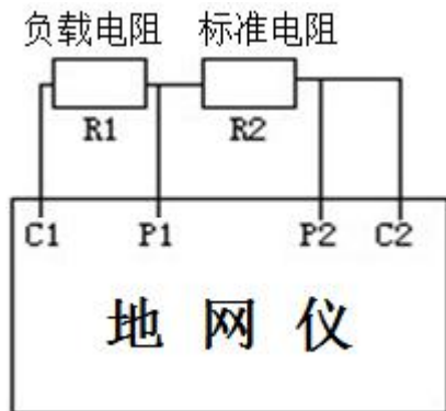
图 1：串入负载电阻后的接线图
