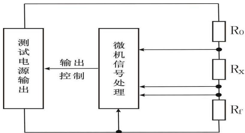
图 1 测量原理示意图
