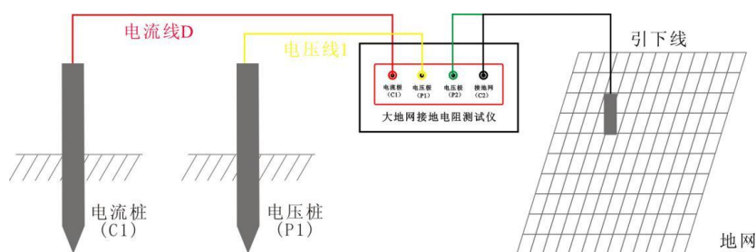
图3 三极法测量接线图
