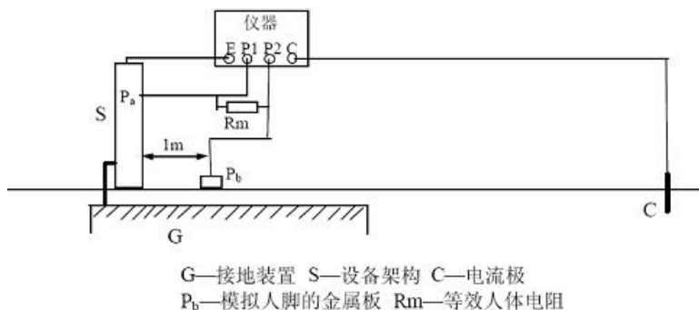
图5 接触电压测量接线图
