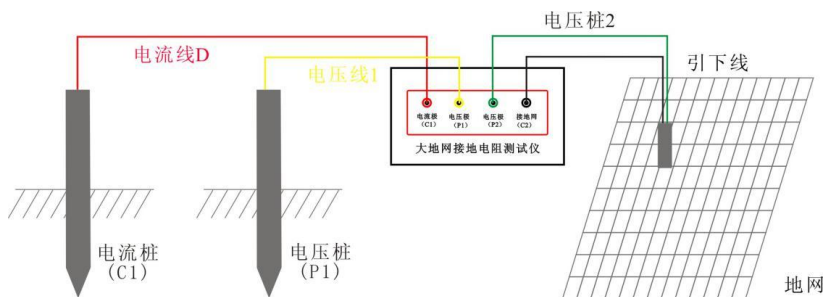
图4 四极法测量接线图
