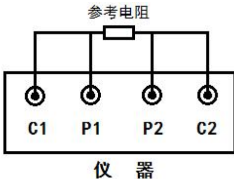
图 13 仪器自检接线图
