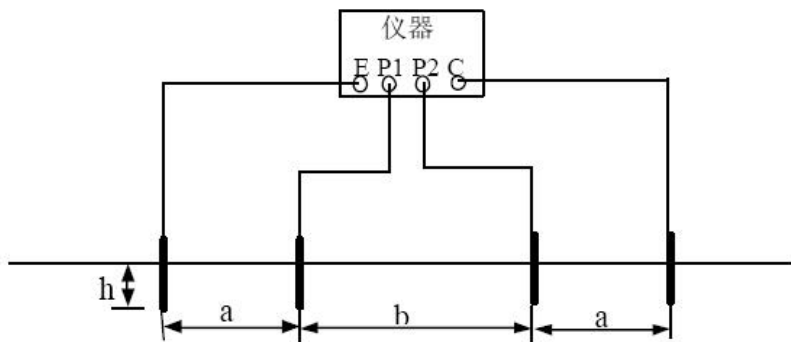
图7 四极法测量土壤电阻率接线图
